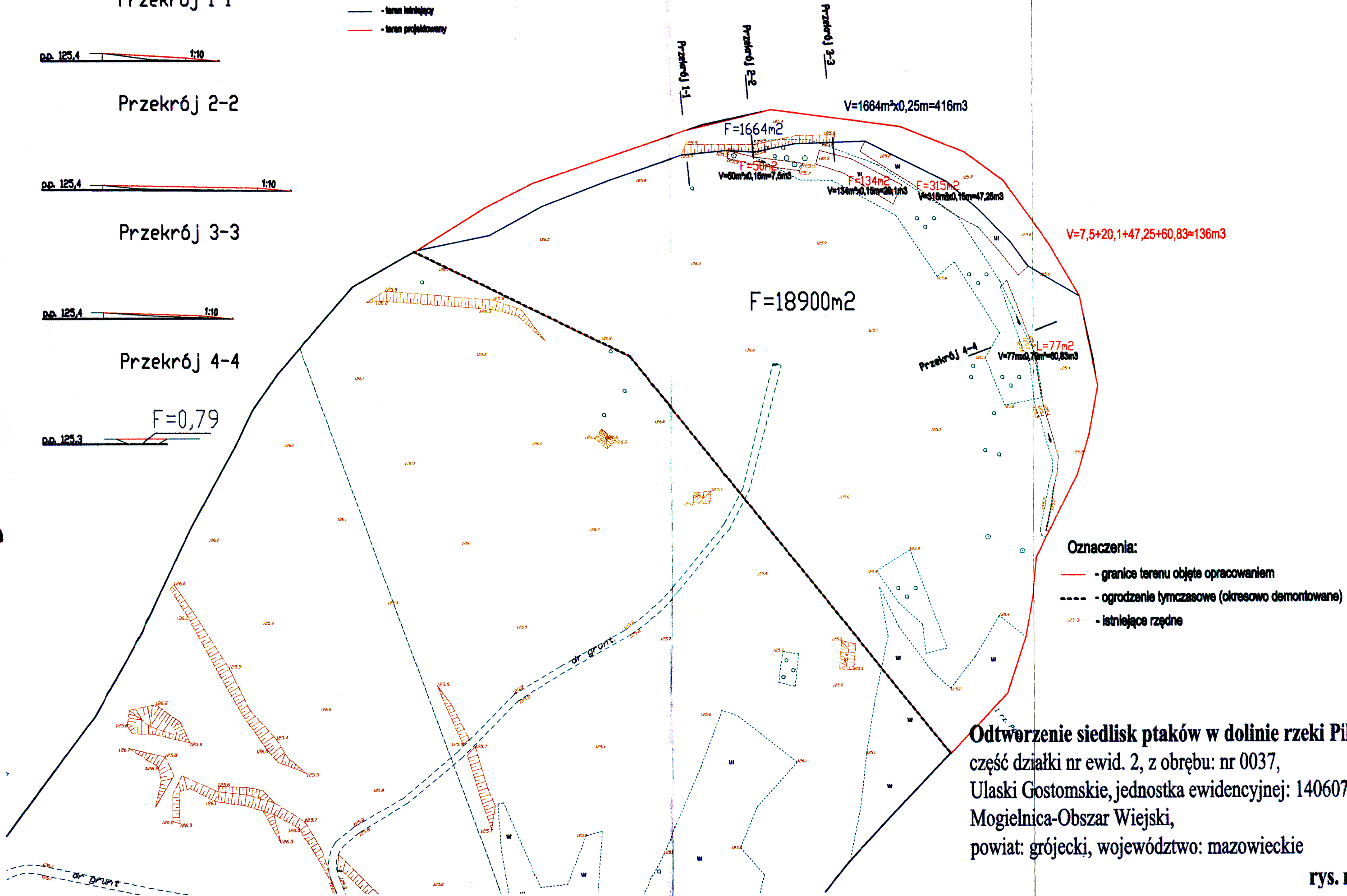
Przekrój 1-1
