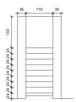
ELEWACJA WSCHODNIA INWENTARYZACJA
