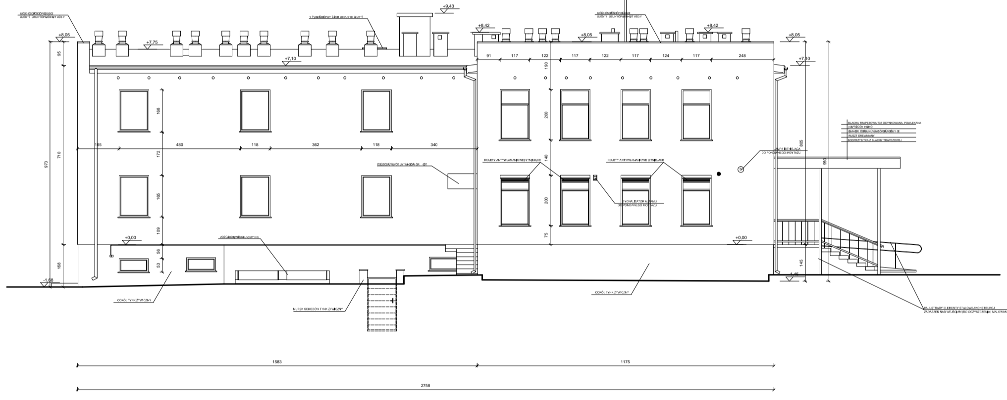
ELEWACJA WSCHODNIA
