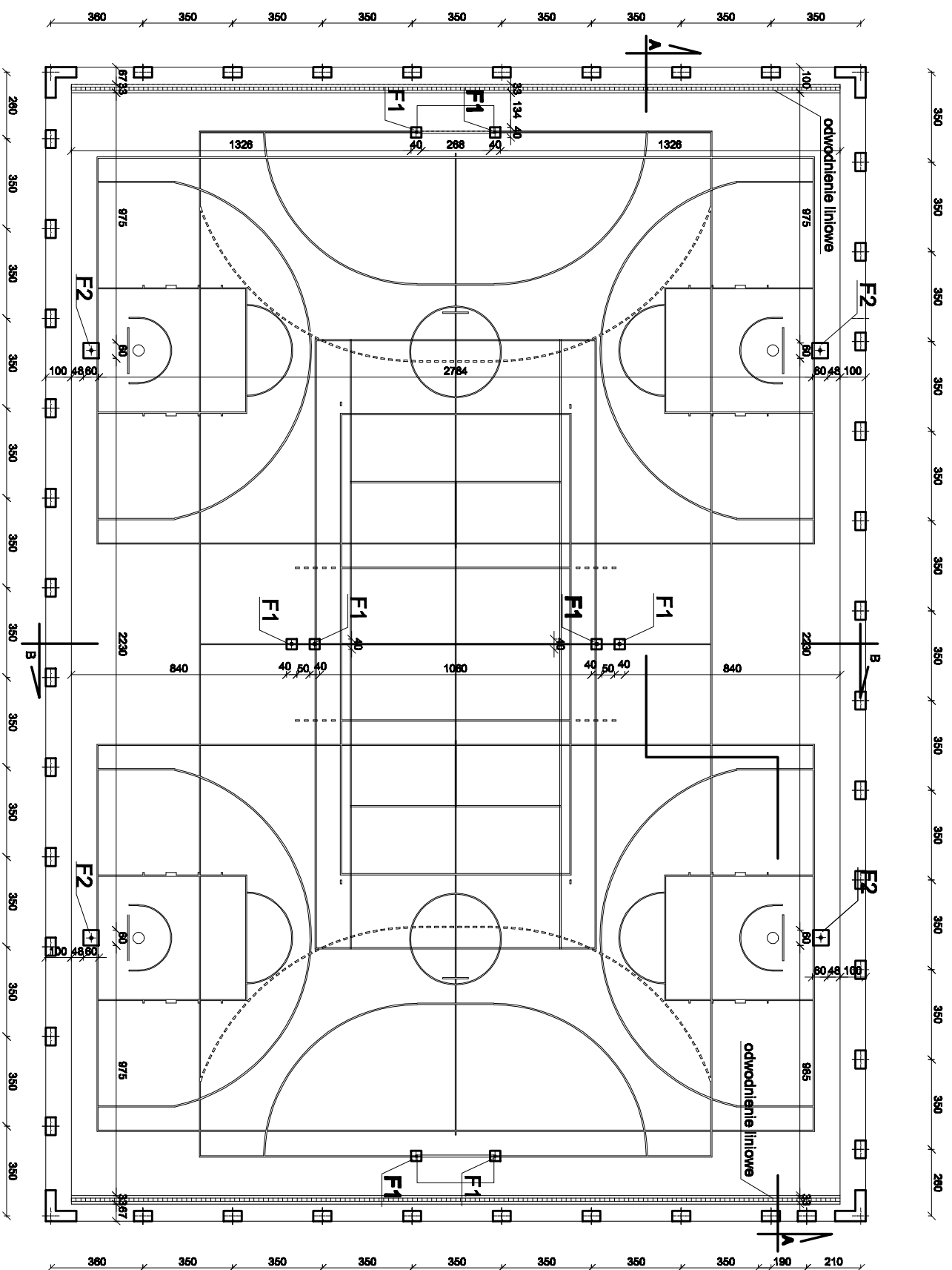
FUNDAMENT F2
